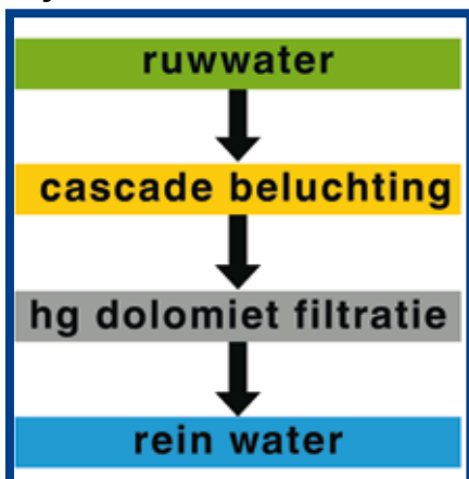
Afb. 6: Proces van een pompstation met filtratie over halfgebrande dolomiet.
