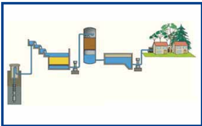
Afb. 2: Processchema van een pompstation met cascadebeluchting, zandfiltratie en torenbeluchting.
